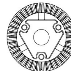
Bevel gear set 36-15 ×2 傘齒組 36-15 310073
